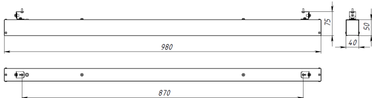
Рисунок 3 - Габаритные размеры при комплектации с креплением уголок на примере Line 980мм.
